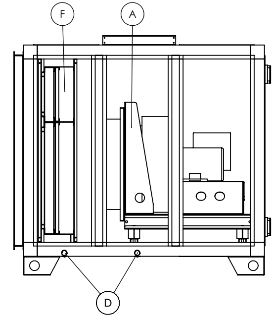
Perspektif/Perspective
