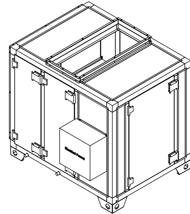
Perspektif/Perspective
